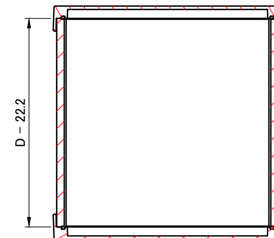
C-C ( 1 : 3.5 )
